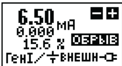
Рисунок 6.4 – Экран прибора в режиме генерации тока с плавным изменением задания
