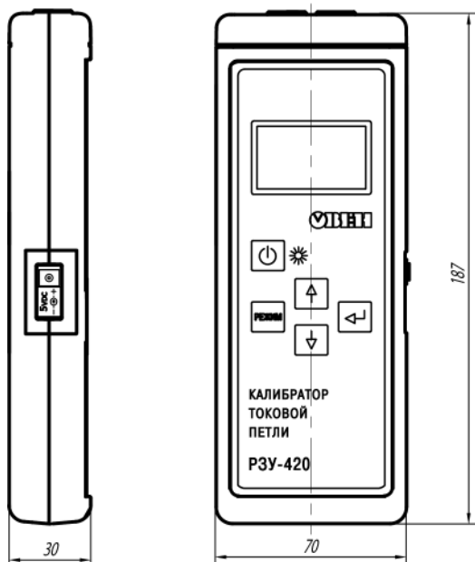
Рисунок А.1 – Габаритный чертеж прибора
